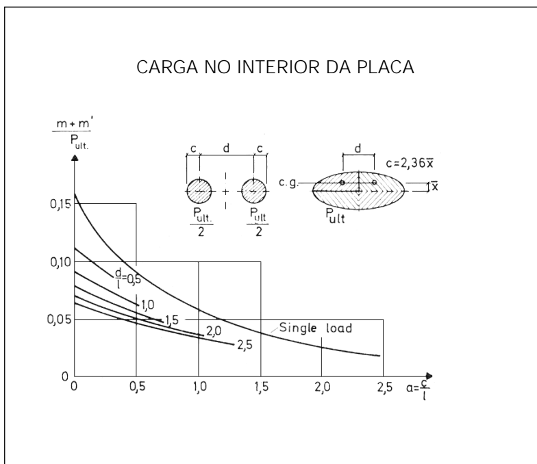
Figura 4 Diagrama de momentos atuantes para carga no interior da placa
