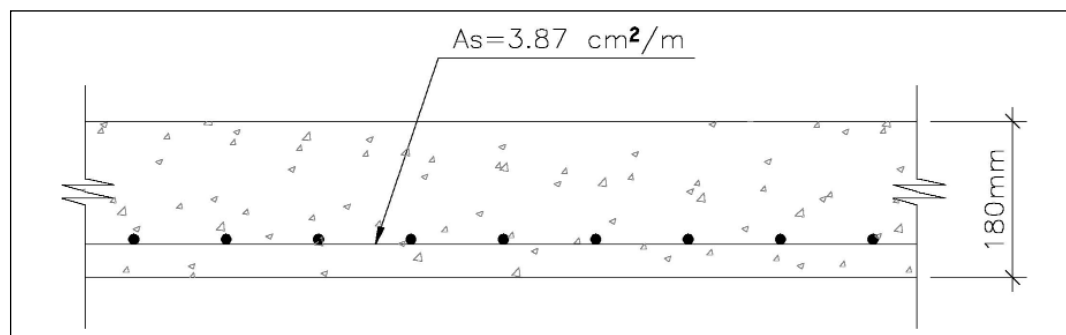
Figura 1 Seção típica do Aeroporto de Estocolmo ( 3 )
