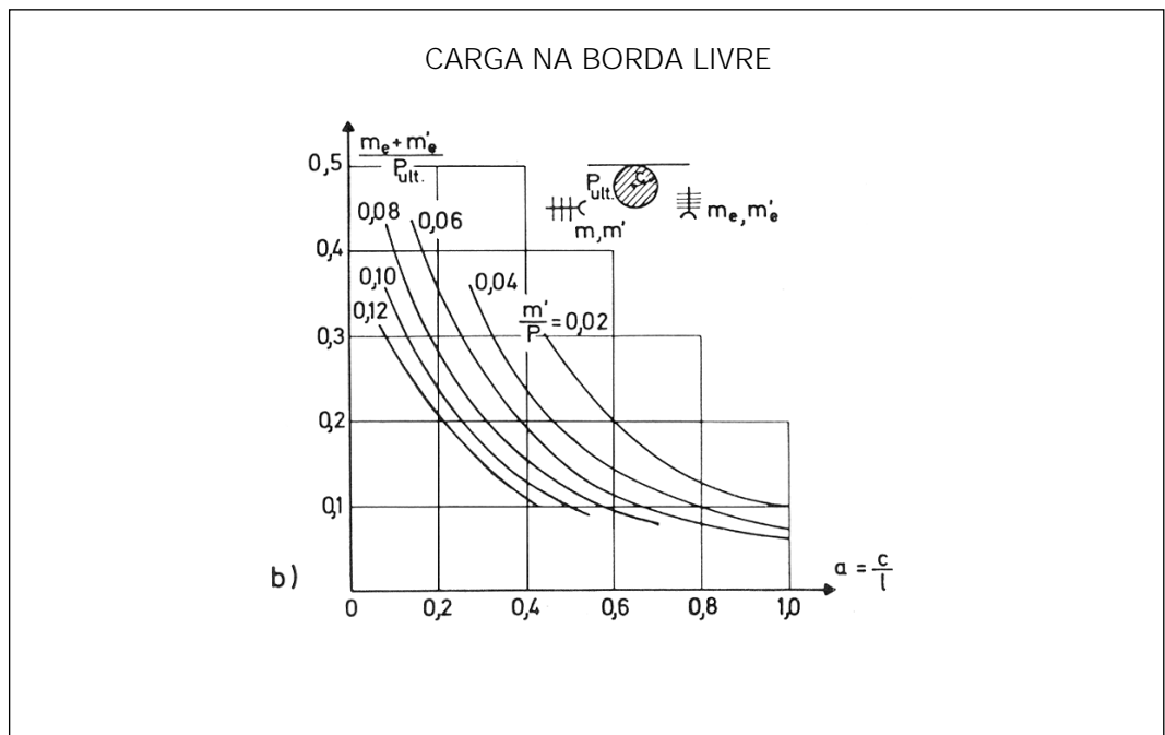
Figura 6 Diagrama de momentos atuantes para carga na borda livre da placa
