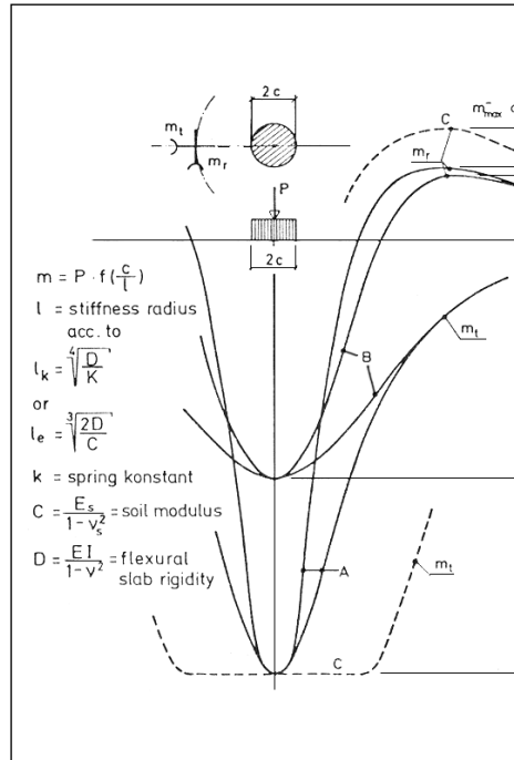
Figura 2 Distribuição aproximada dos momentos fletores
