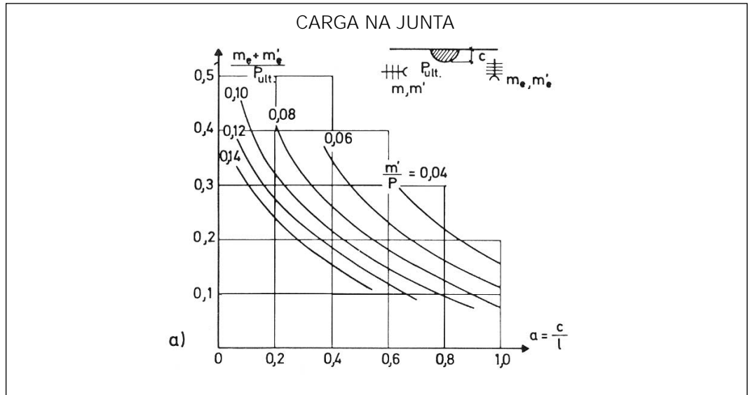
Figura 5 Diagrama de momentos atuantes para carga na junta (com barras de transferência) da placa
